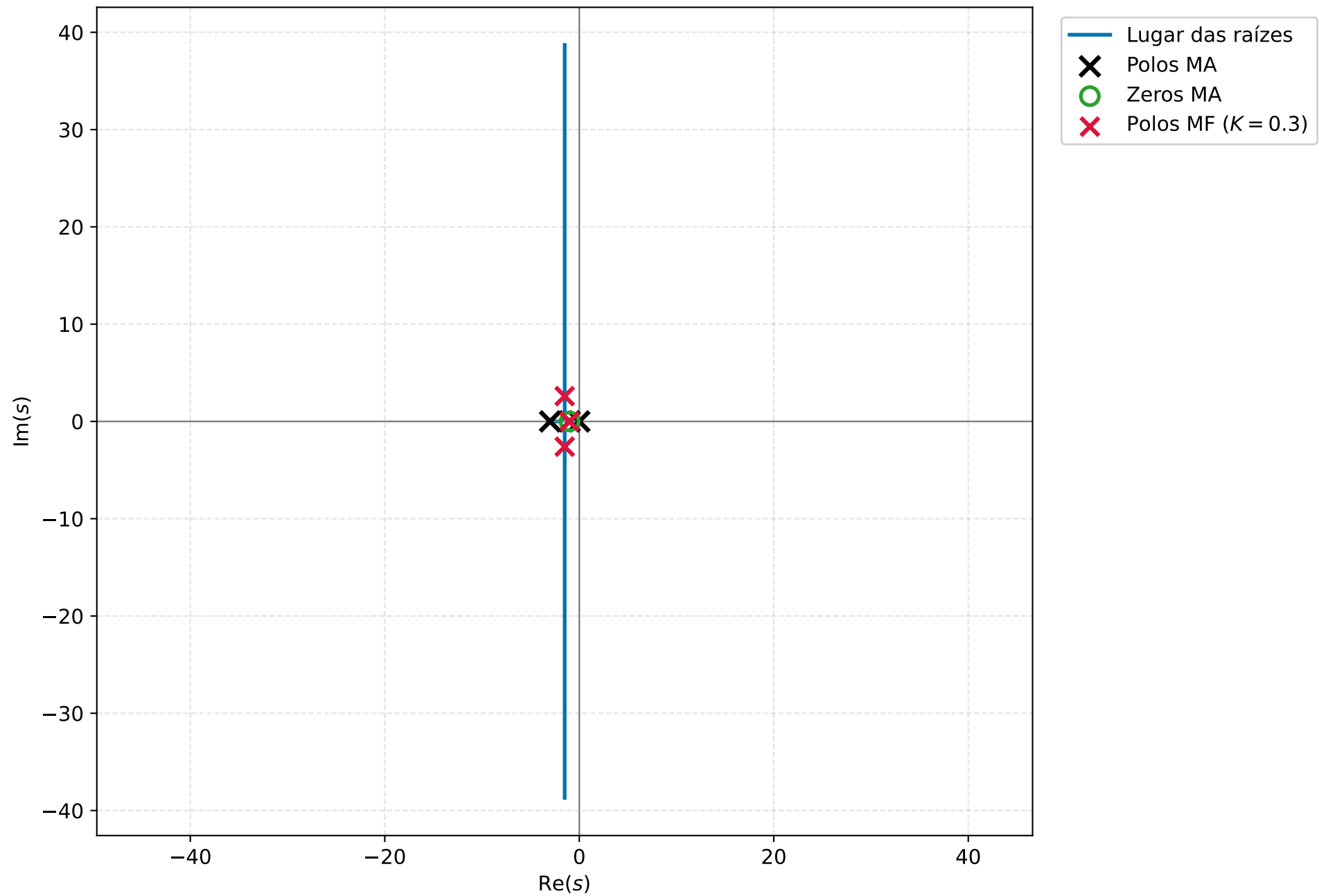
Questão B.6.15 --- LR de \Phi(s) = G(s)/K , malha 1 + K\Phi = 0
